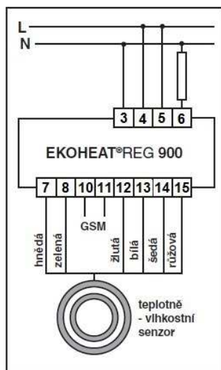
Schéma zapojení regulace EKOHEAT ® REG 900 s čidly pro ochranu venkovních ploch
