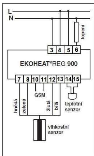
Schéma zapojení regulace EKOHEAT ® REG 900 s čidly pro ochranu okapů.
